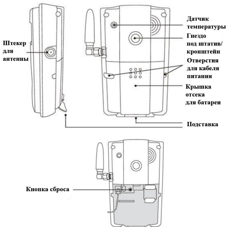
Рисунок 1. Элементы камеры
