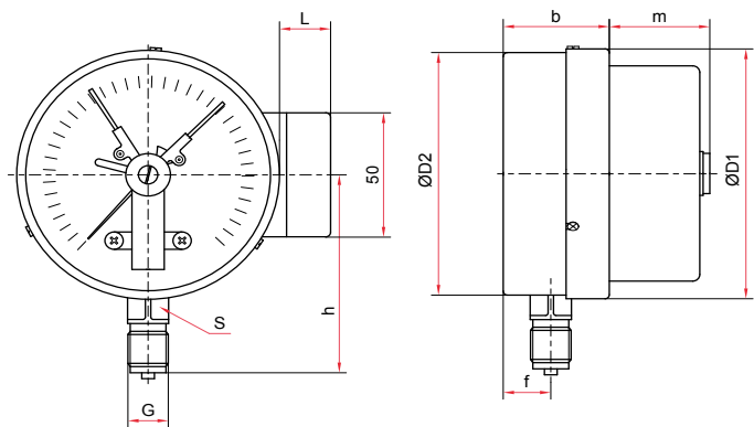
Радиальное присоединение
