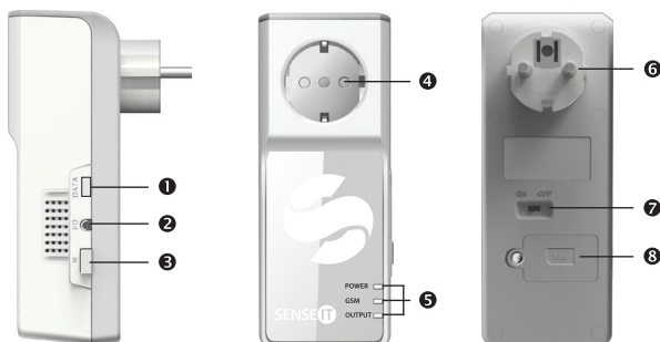
Рис. 1: Внешний вид умной розетки
