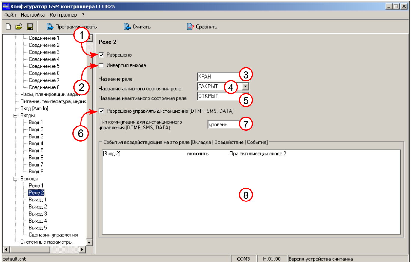
Рисунок 17. Параметры реле 2 для управления краном НР12В
